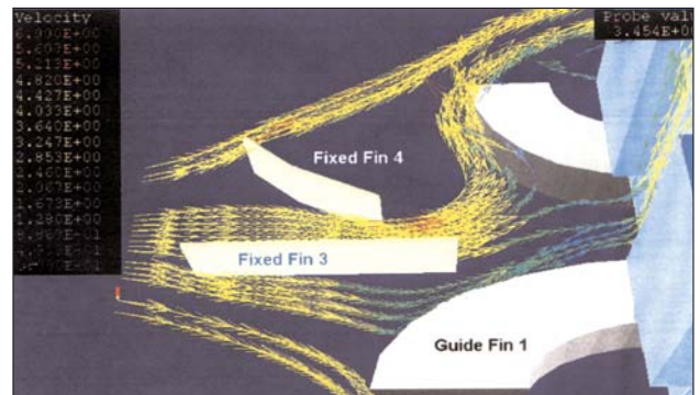
Option 2a - Two Guide Fins
